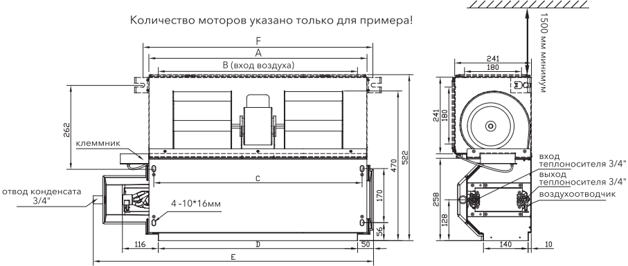
Габаритные размеры, мм
