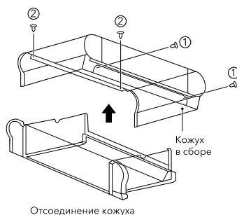
Отсоединение кожуха
