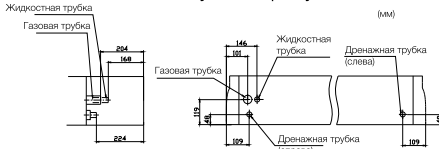
Положения соединений труб
