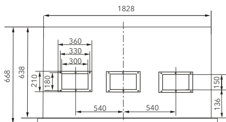
Схема расположения отверстий под соединительные винты выпускного воздуховода. EACD-150HWN1 IN
