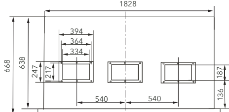
Схема расположения отверстий под соединительные винты подающего воздуховода. EACD-192HWN1 IN
