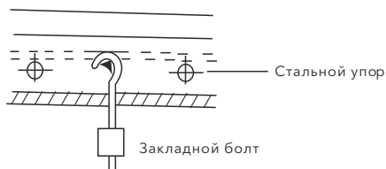
Закладной болт для подвешивания трубы
