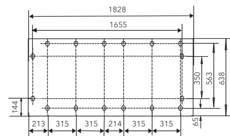
Схема расположения отверстий под винтовые винты заборного воздуховода.
