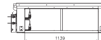
Схема расположения отверстий под соединительные винты подающего воздуховода.
