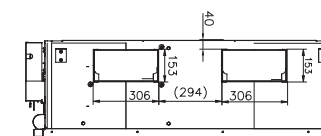
Схема расположения отверстий под соединительные винты выпускного воздуховода.
