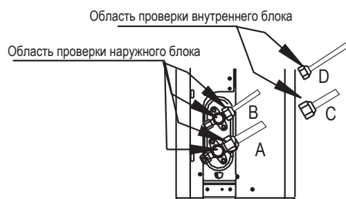
A: Запорный вентиль низкого давления B: Запорный вентиль высокого давления C & D: Конусные гайки внутреннего блока
