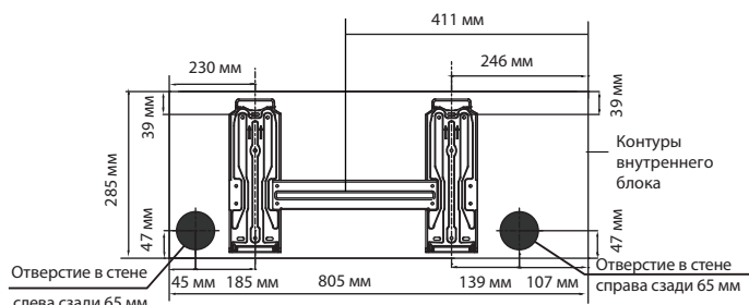
РК-12SDM4
