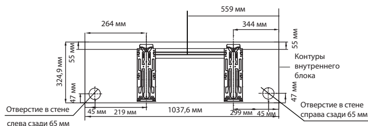
РК-24SDM4
