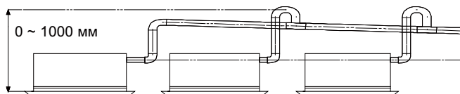
Тройники, объединяющие дренажные трубопроводы
