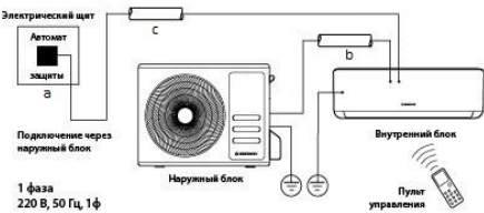
Блок - схема подключения кондиционера к однофазной сети
