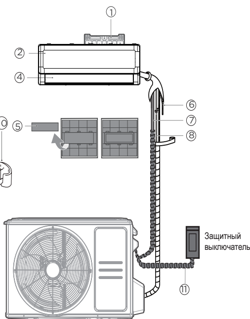
Модели с электропитанием от наружного блока
