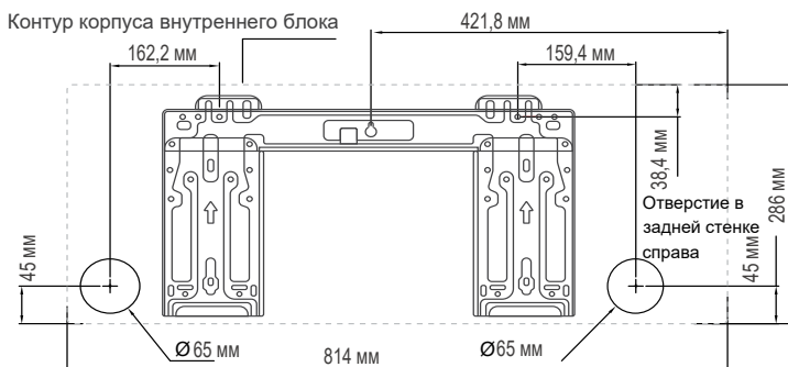
Типоразмер 12K
