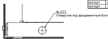
ВидА
