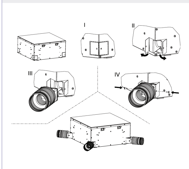
» Obr. 17 FWH-A 02-03-04
