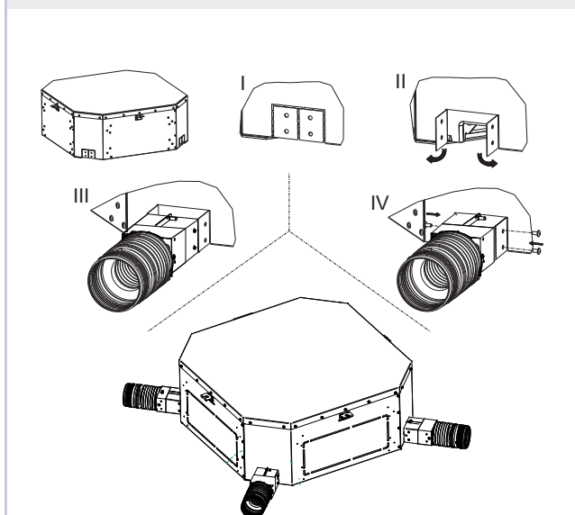
» Obr. 18 FWH-A 06-07-08
