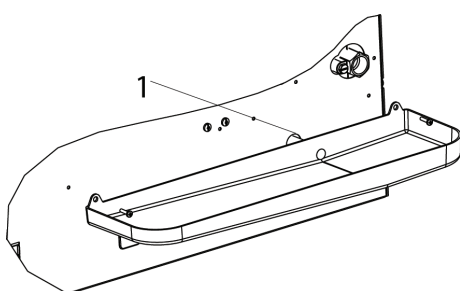
1 Scarico condensa
