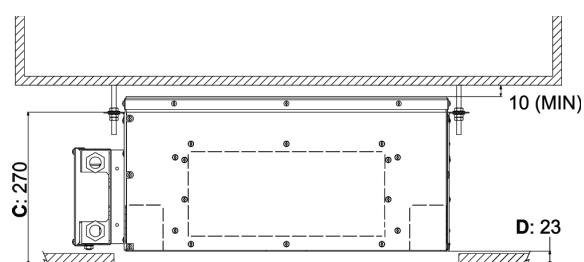
» Abb.9 FWH 02-03-04
