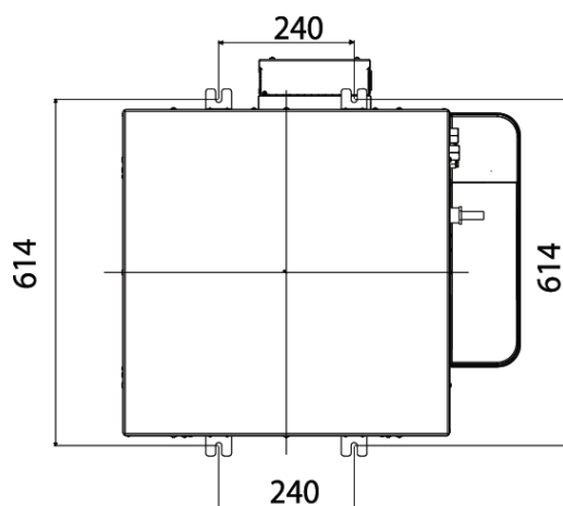
» Abb.4 FWH 02-03-04
