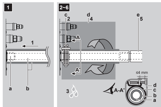
а Соединение сливного трубопровода (с блоком) б Сливной шланг (в комплекте принадлежностей) в Металлический зажим (в комплекте принадлежностей) г Уплотнительная подушка большого размера (в комплекте принадлежностей) е Сливной трубопровод (приобретается по месту установки)
