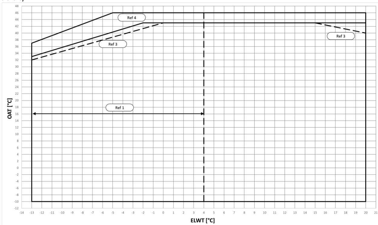
Рис. 1. Эксплуатационные пределы EWYTx5B-S в режиме охлаждения
