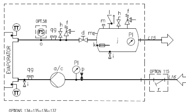
Рис. 16. Гидравлическая схема для одного насоса / двух насосов с баком (EWYTxh5B) (компл. 134-135) (макс. рабочее давление 6 бар)
