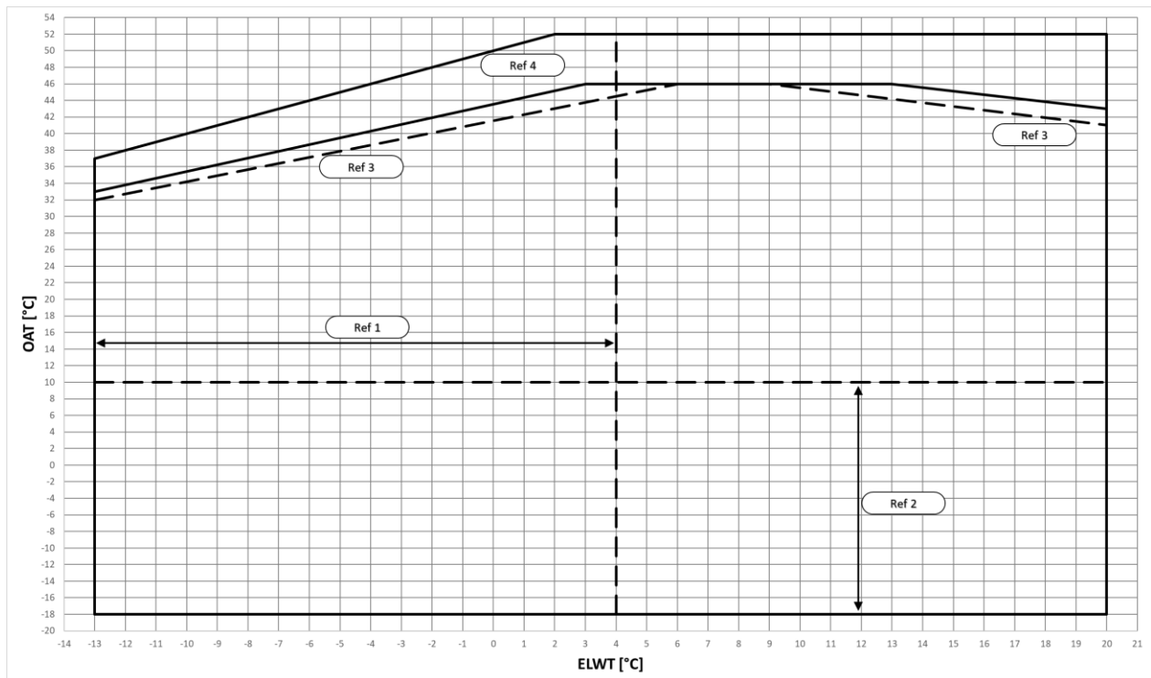
Рис. 3. Эксплуатационные пределы EWYTx0B-S в режиме охлаждения
