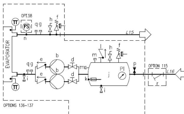
Рис. 17. Гидравлическая схема для сдвоенного насоса (EWYTxh5B) (компл. 80-81/136-137) (макс. рабочее давление 6 бар)
