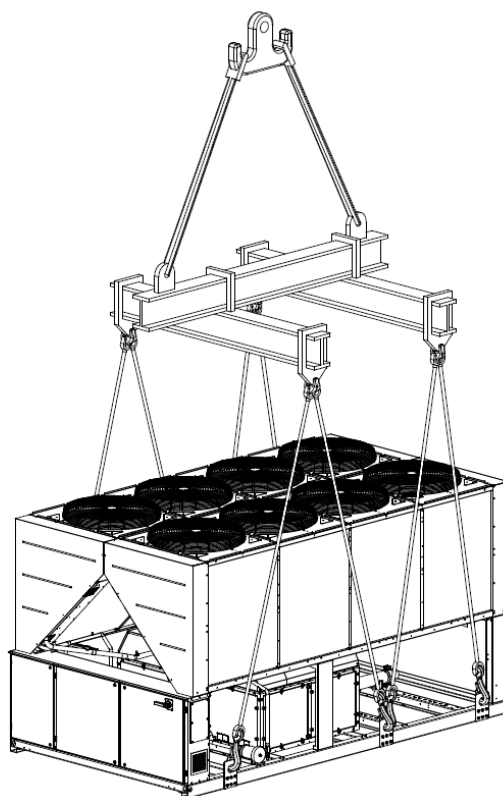
Агрегат с 6 такелажными точками
