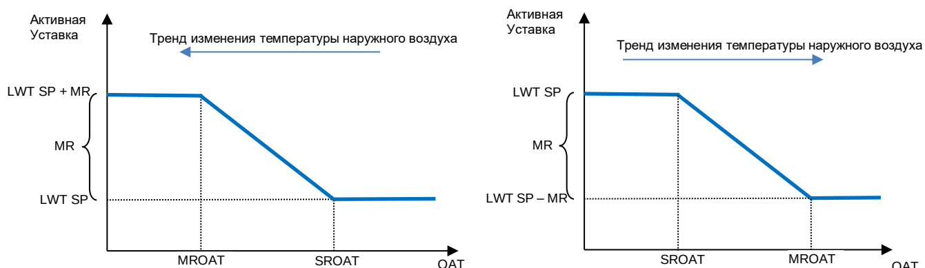
График 2. Зависимость активной уставки от температуры внешней среды.
