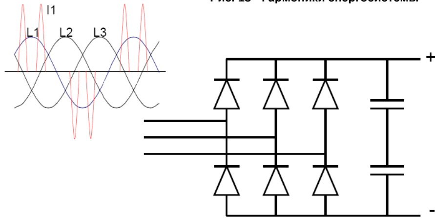
Рис. 13 - Гармоники энергосистемы
