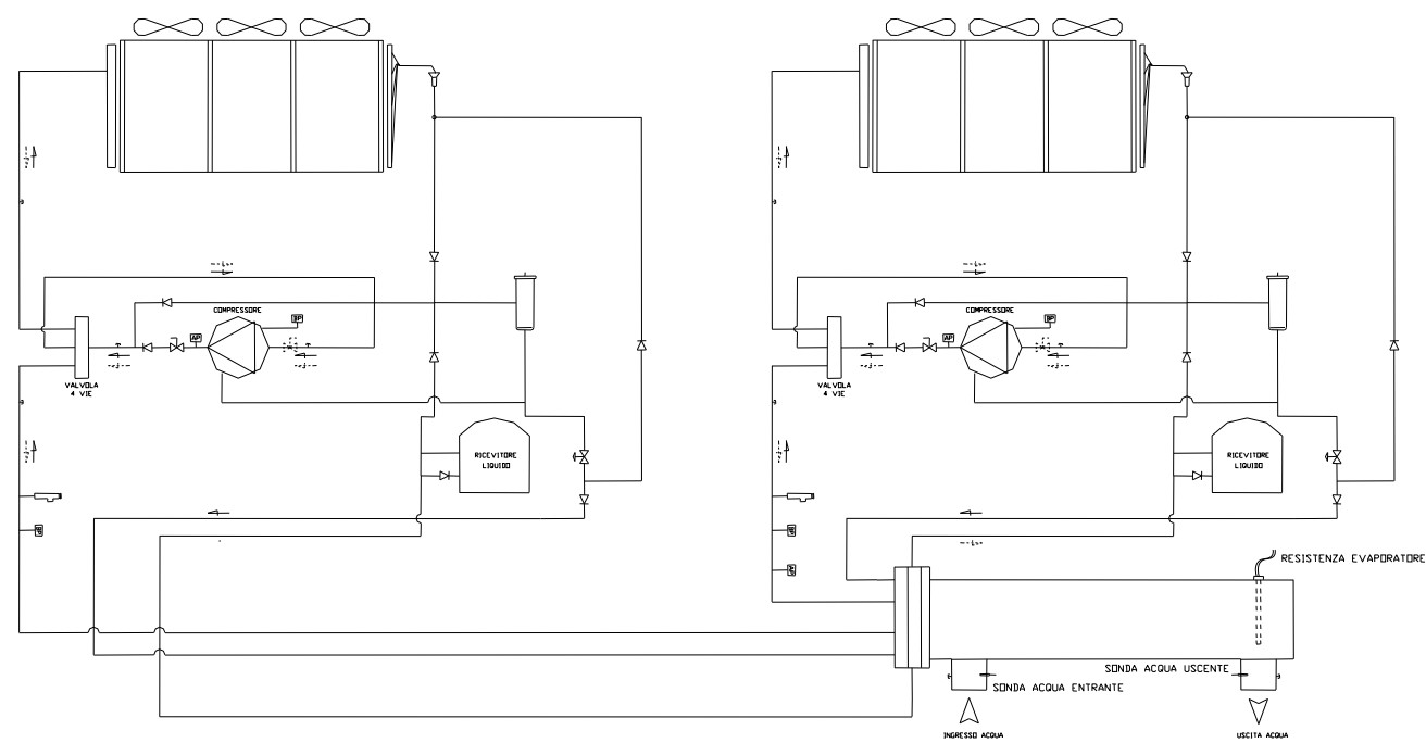
Рис. 16 - Холодильный цикл
