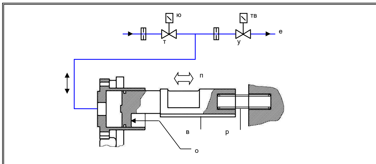
Рис. 20 - Механизм управления производительностью компрессора Fr3100
