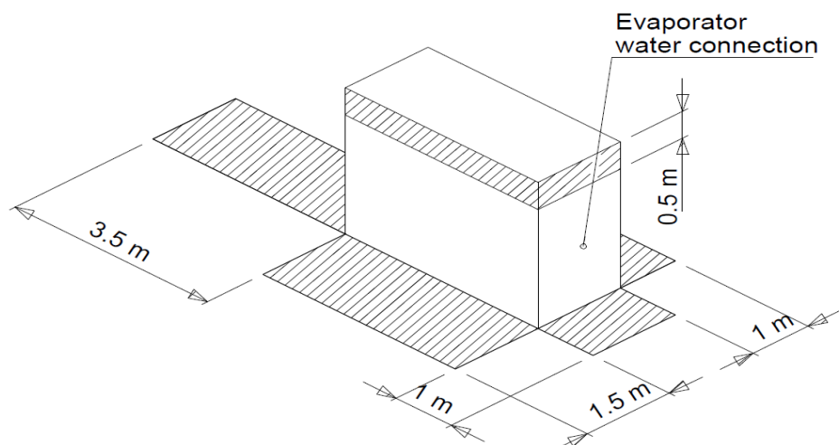
Рис. 9 - Расположение агрегата
