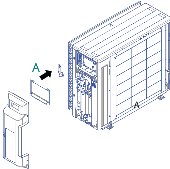
Разборка блока
