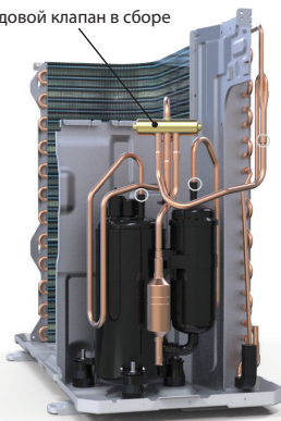
4-ходовой клапан в сборе
