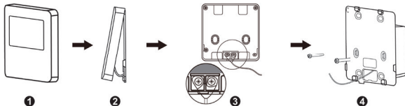
Рисунок 4.9 Демонтаж проводного пульта управления
