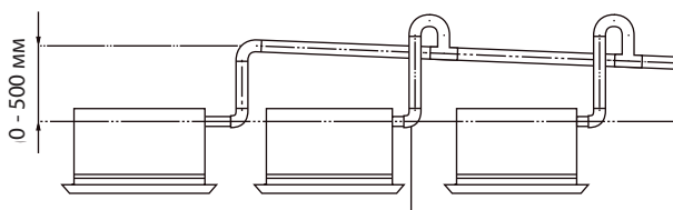
Подключение дренажных трубок с помощью тройников
