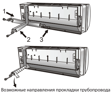
Возможные направления прокладки трубопровода
