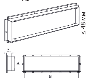
Рис. 6. Воздуховыпускное отверстие
