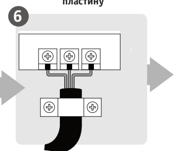
Подключите электропроводку
