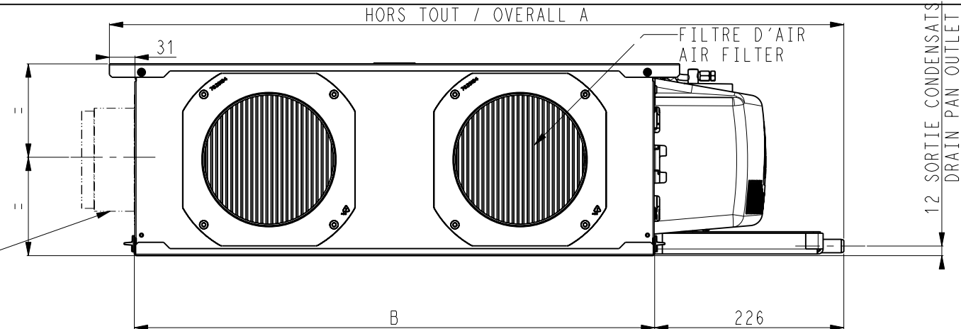
VUE FACE AU SOUFFLAGE FRONT VIEW AIR SUPPLY
