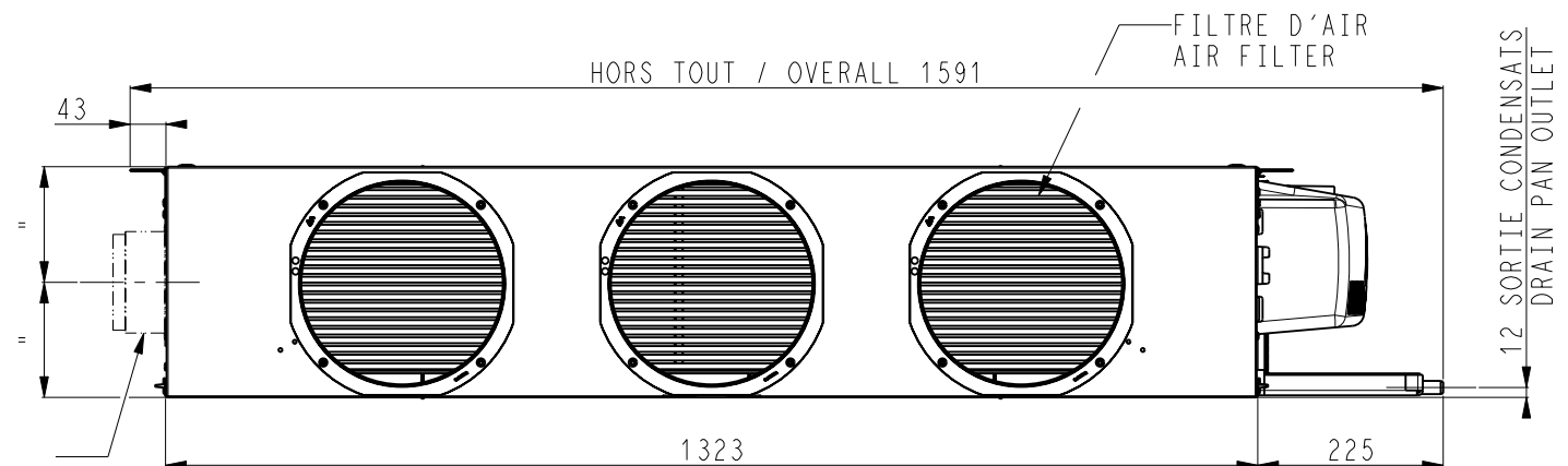
42NX T5 VUE FACE AU SOUFFLAGE FRONT VIEW AIR SUPPLY
