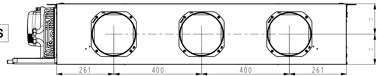
VIROLES / SPIGOTS Ø200
