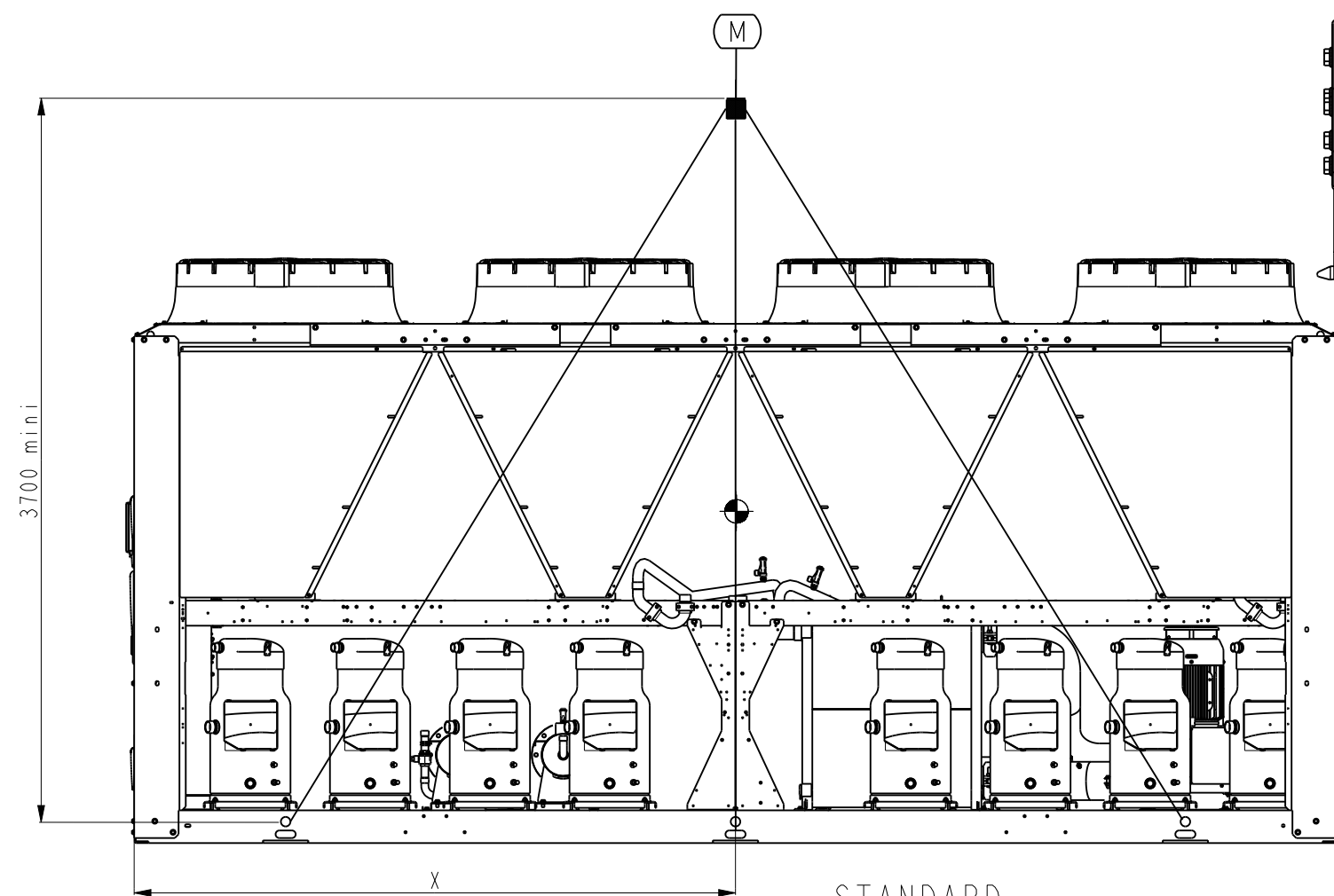
DETAIL G Echelle 9:64
