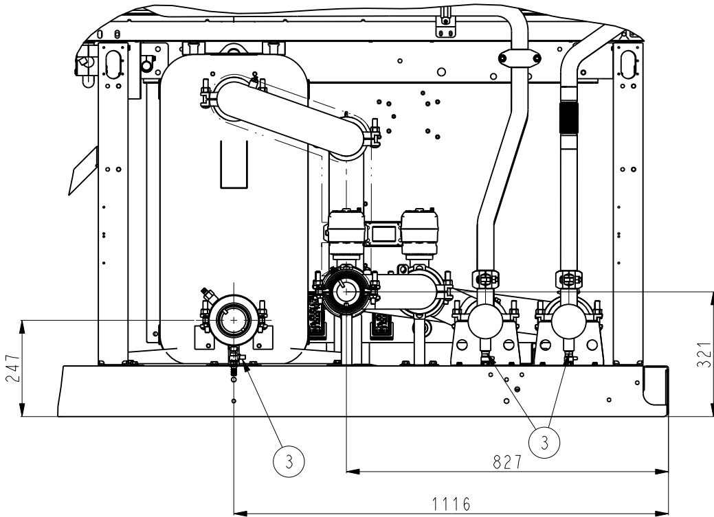
VUE / VIEW H ECHELLE 3:40
