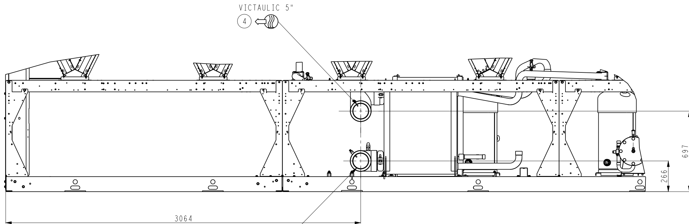
ECHELLE 1:20
