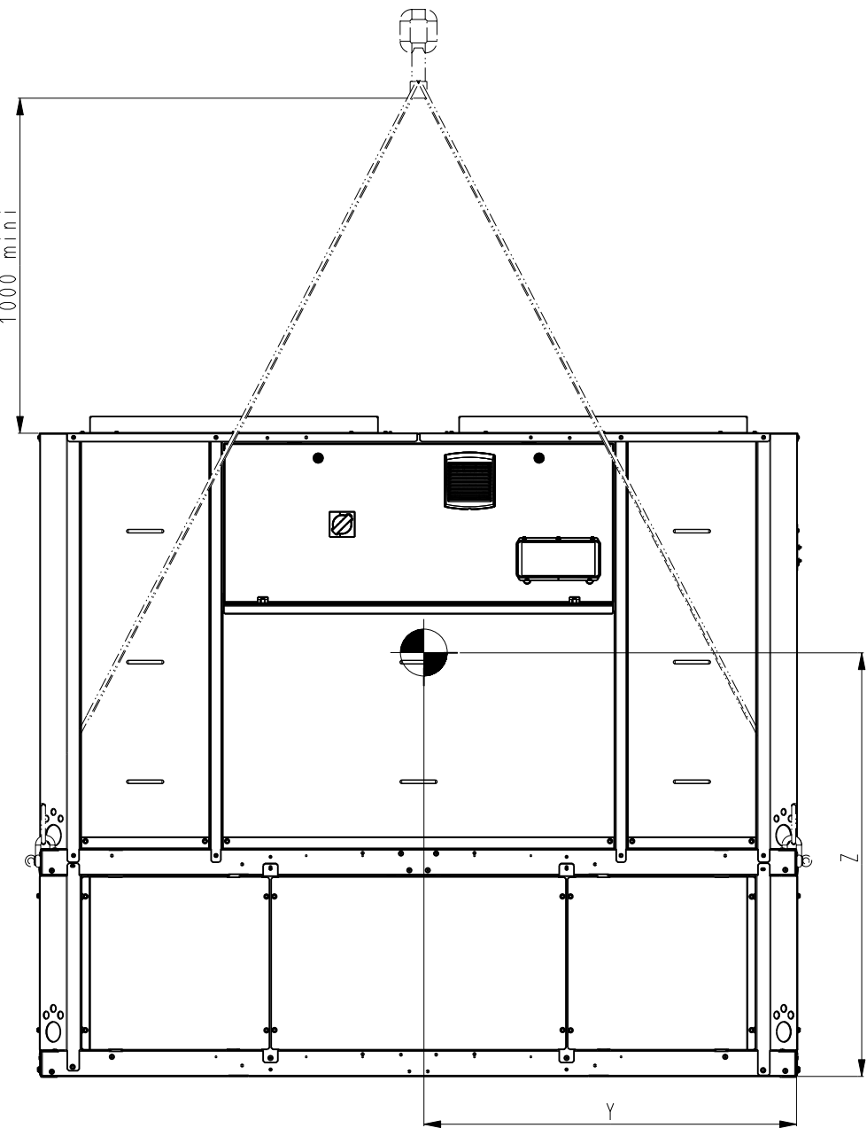
COUPE / SECTION B-B ECHELLE 5:16
