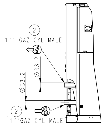
DETAIL FOR 2 DETAIL POUR 2 PLACES
