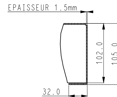
DETAIL S ECHELLE 1:4
