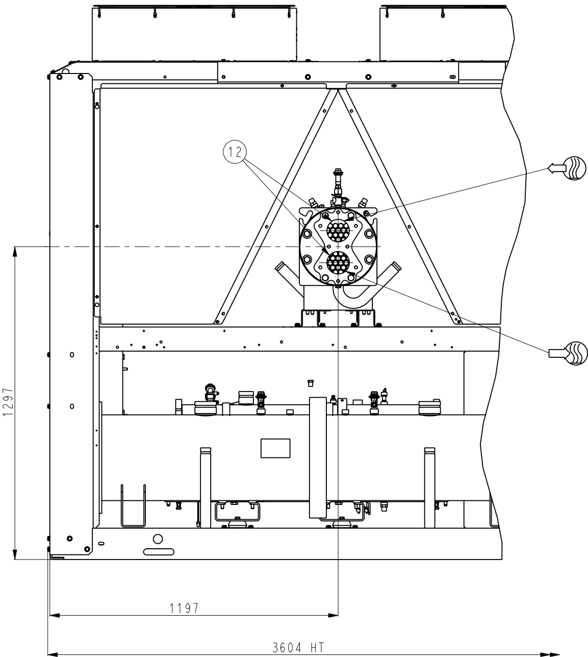
VUE F ECHELLE 1:16
