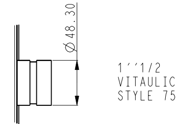
DETAIL A Echelle 1:4
