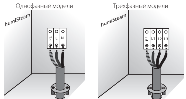
Рис. 4.c (вид внутри агрегата, электрическая секция)
