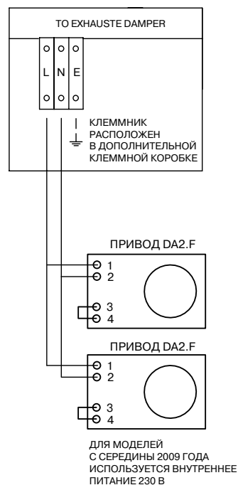
СИСТЕМА ЗАЩИТЫ ОТ ЗАМОРАЖИВАНИЯ DELTA 1-16
