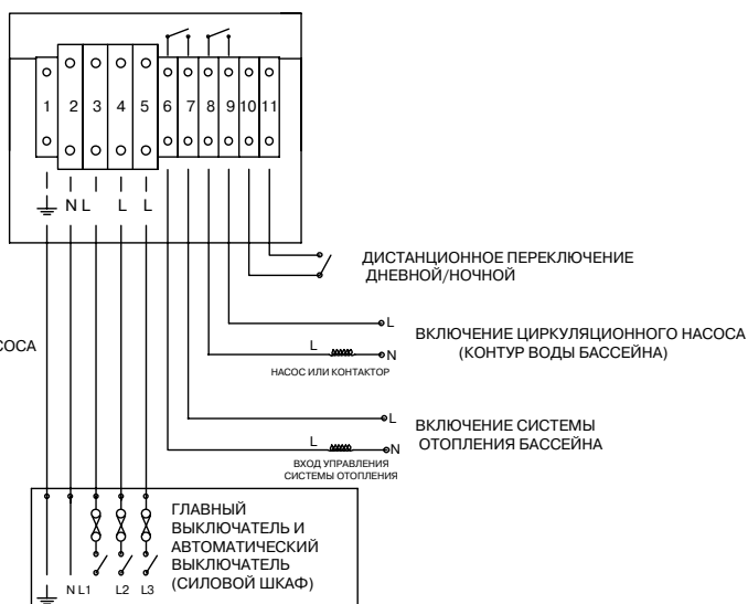
DELTA 1-12 (ТРЕХФАЗНЫЕ МОДЕЛИ) ОСНОВНОЙ КЛЕММНИК
