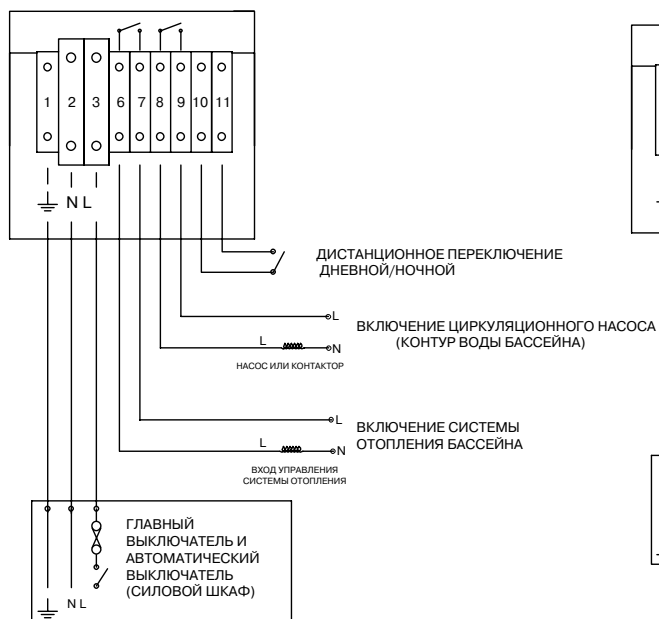
DELTA 1-6 (ОДНОФАЗНЫЕ МОДЕЛИ) ОСНОВНОЙ КЛЕММНИК
