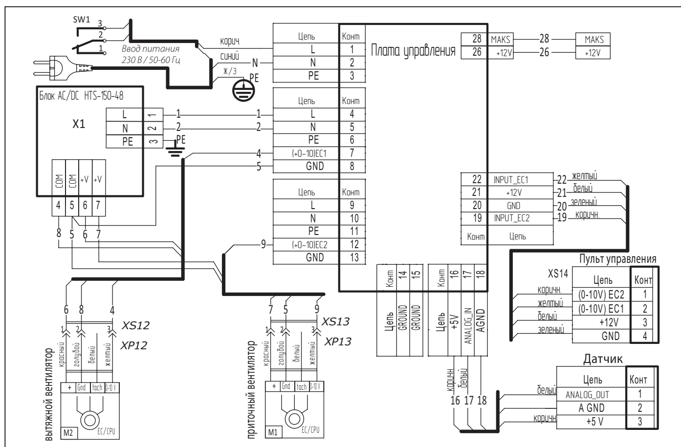
Рис. 6. Электрическая схема установки
