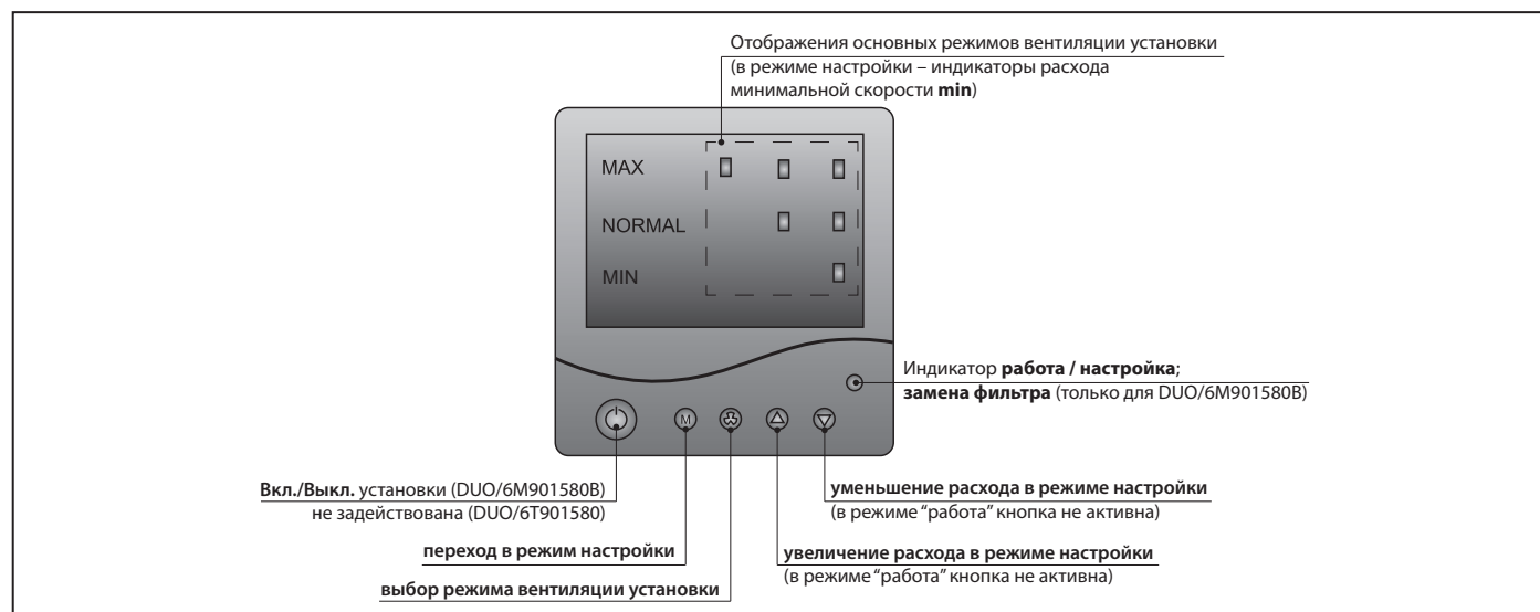
Рис. 7. Панель управления
