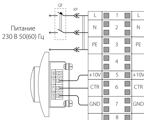
Схема внешних подключений для автоматики S2
