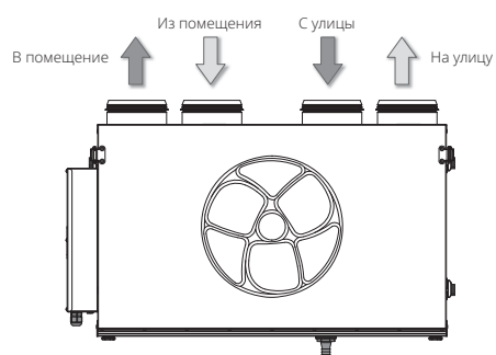
Komfort Ultra (EC) L 250 (300)-H(E) — левое исполнение
