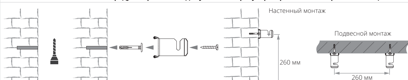
Настенный монтаж при помощи монтажных кронштейнов
