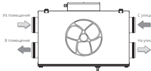
Komfort Ultra (EC) L 250 (300)-H(E) — левое исполнение
