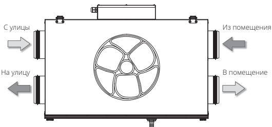
Komfort Ultra (EC) L 250 (300)-H(E) — правое исполнение
