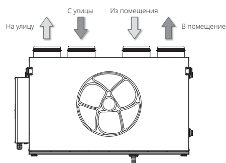
Komfort Ultra (EC) L 250 (300)-H(E) — правое исполнение
