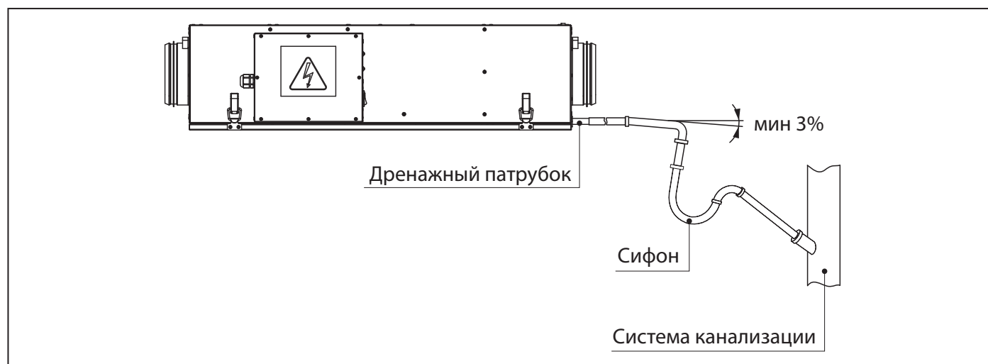
Рис. 5. Отвод конденсата для KOMFORT Ultra Duo D220-H
