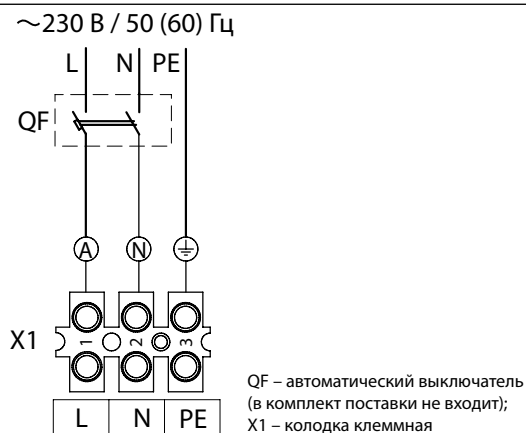
Рис. 7. Схема подключения питания установки
