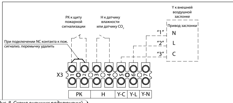
Рис. 8. Схема внешних подключений
