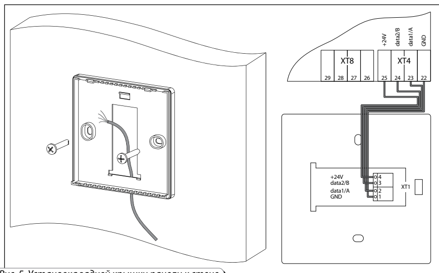
Рис. 5. Установка задней крышки панели к стене
