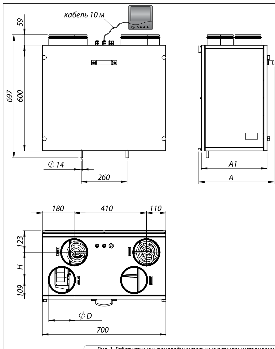
Рис. 1. Габаритные и присоединительные размеры установки
