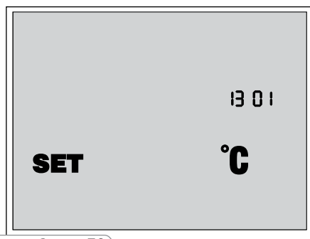
Рис. 15. Версия ПО
