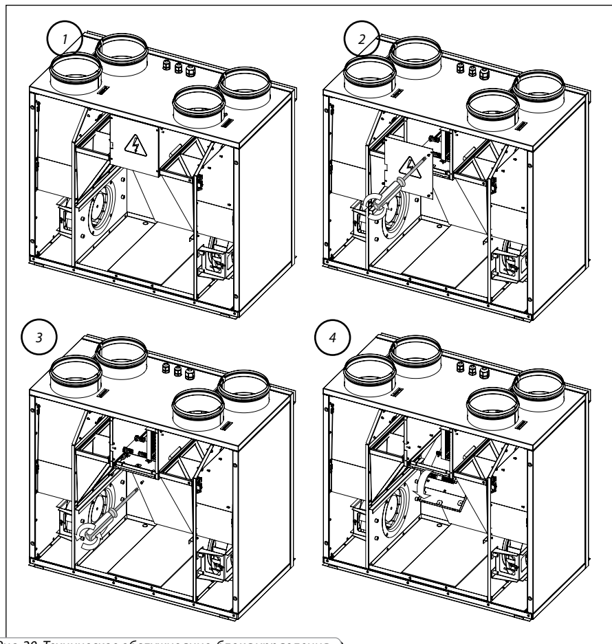
Рис. 20. Техническое обслуживание блока управления
