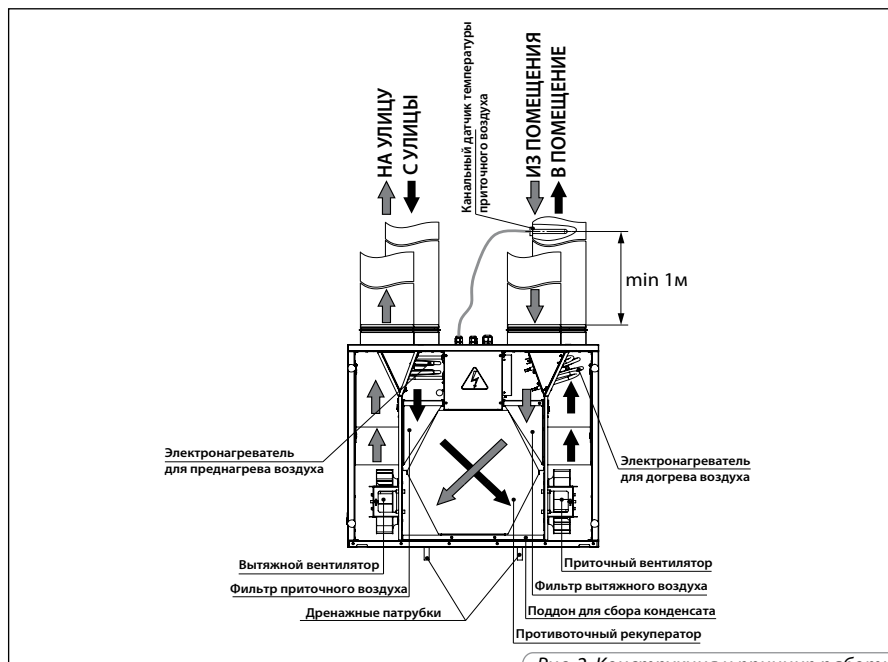
Рис. 2. Конструкция и принцип работы
