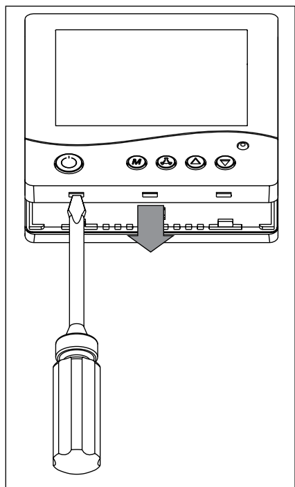
Рис. 4. Отделение задней крышки
