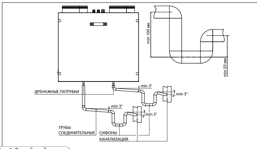
Рис. 6. Отвод конденсата
