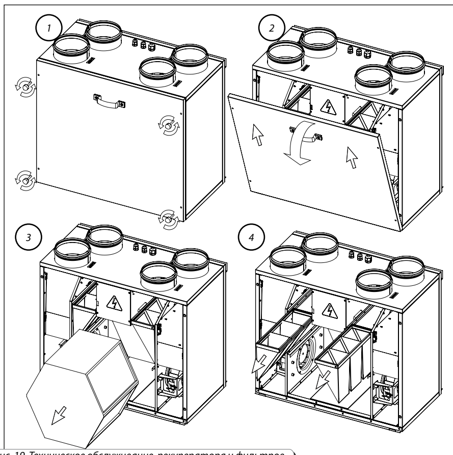
Рис. 19. Техническое обслуживание рекуператора и фильтров
