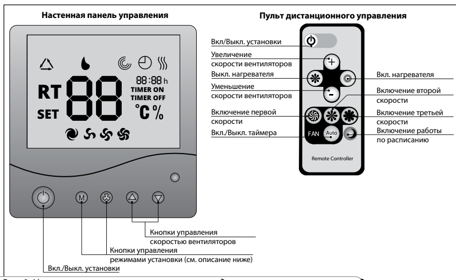
Рис. 9. Настенная панель управления и пульт дистанционного управления
