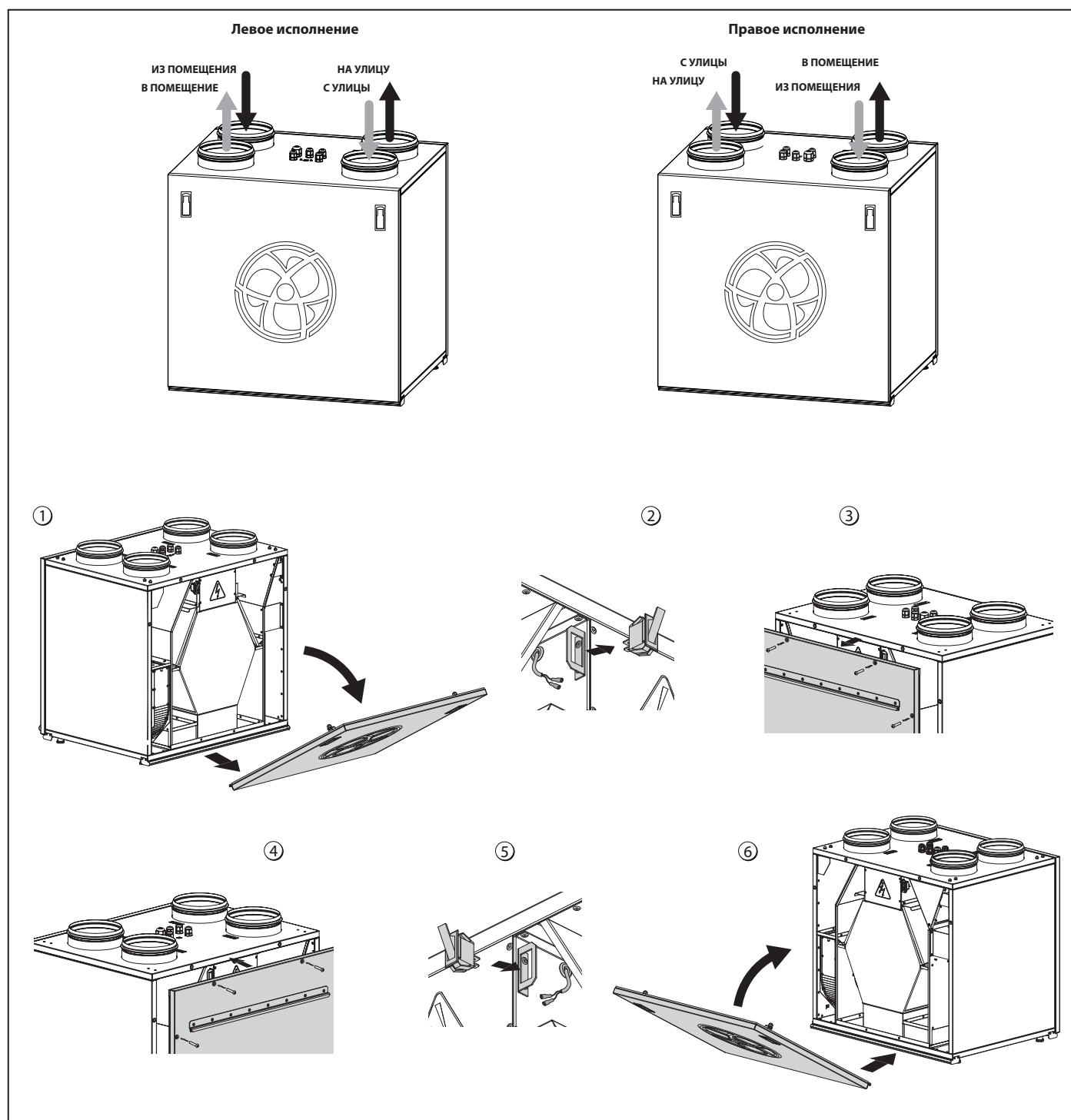
Рис. 12. Сторона обслуживания установки и порядок ее смены
