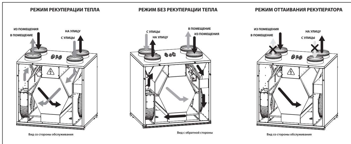
Рис. 2. Режимы работы
