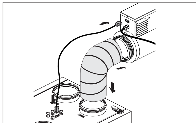
Рис. 12. Монтаж нагревателя
