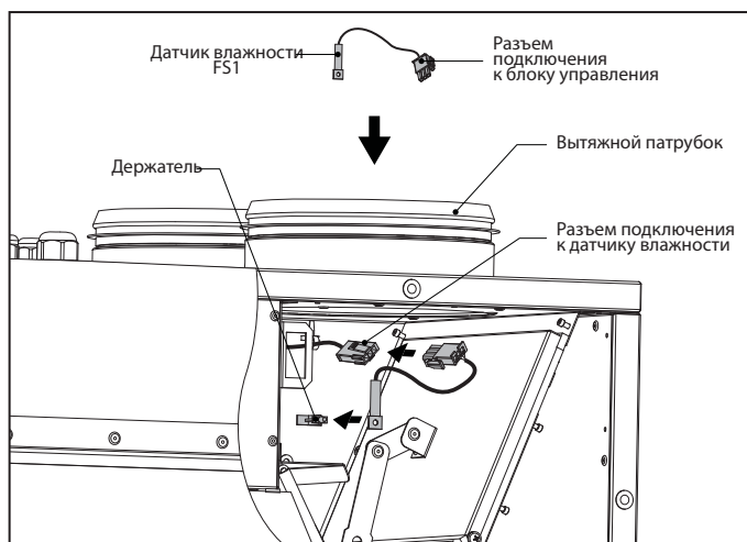
Рис. 10. Монтаж датчика влажности FS1
