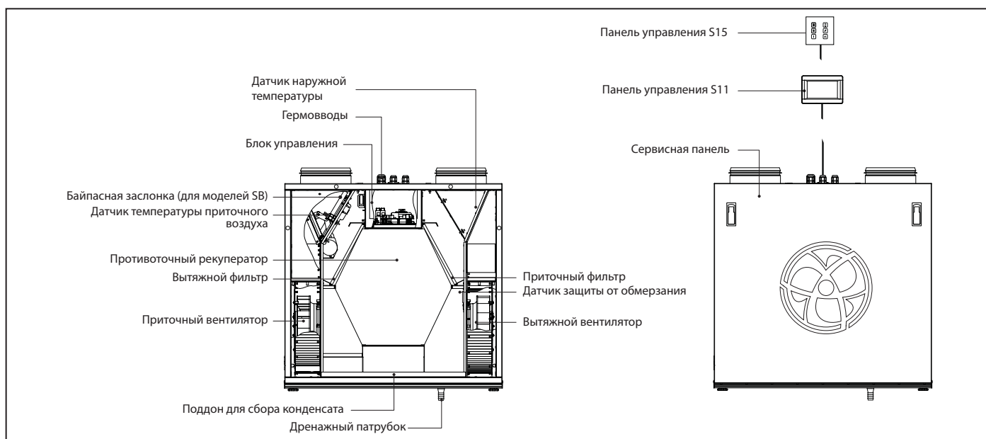
Рис. 1. Устройство установки
