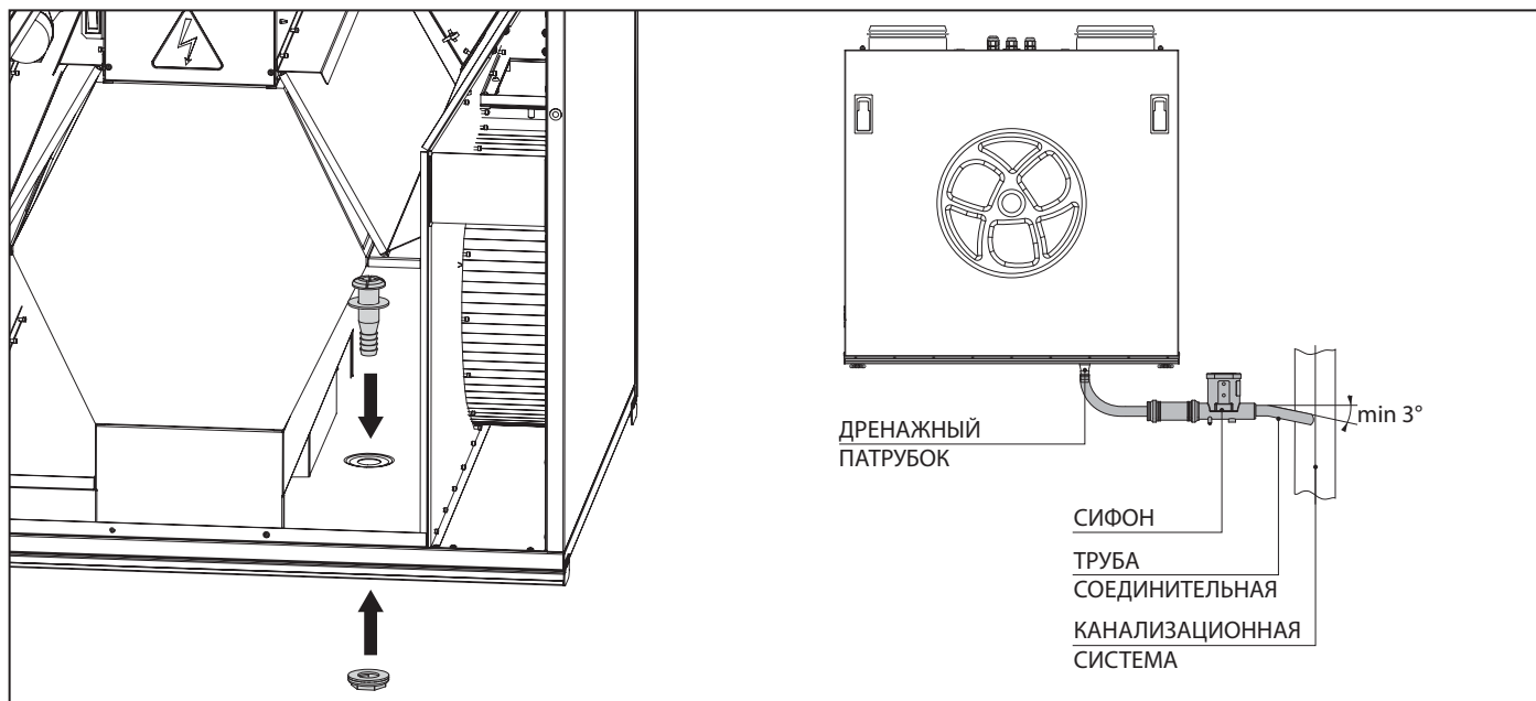
Рис. 16. Отвод конденсата
