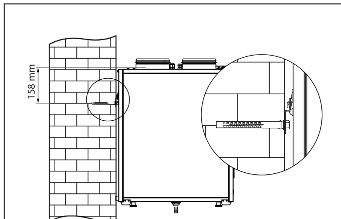
Рис. 8. Настенный монтаж
