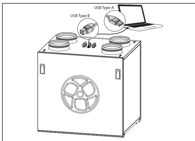
Рис. 21. Подключение ПК к установкам с панелью управления S15
