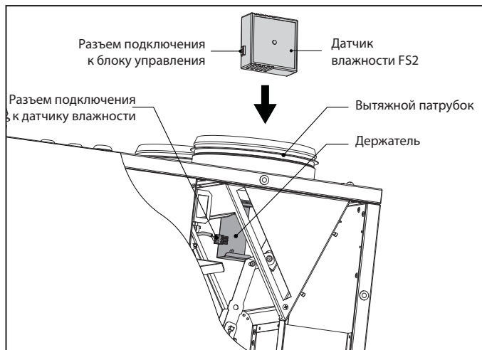
Рис. 11. Монтаж датчика влажности FS2
