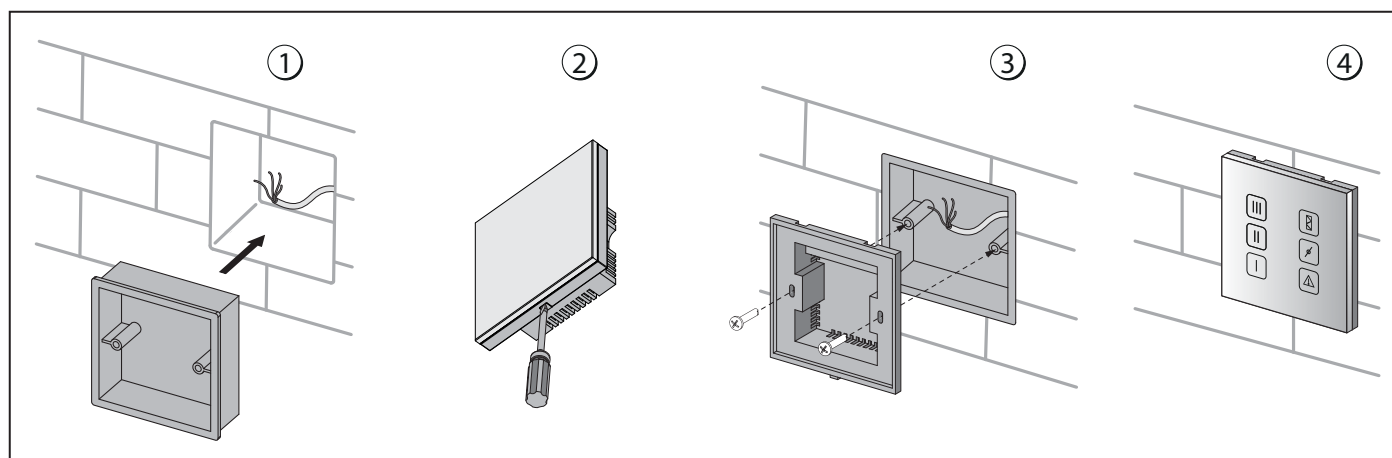
Рис. 14. Внутривентильный монтаж панели управления S15
