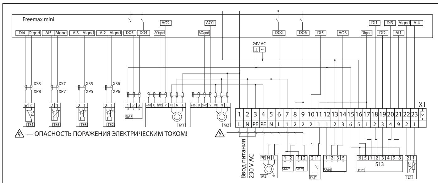
Рис. 10. Схема электрических подключений
