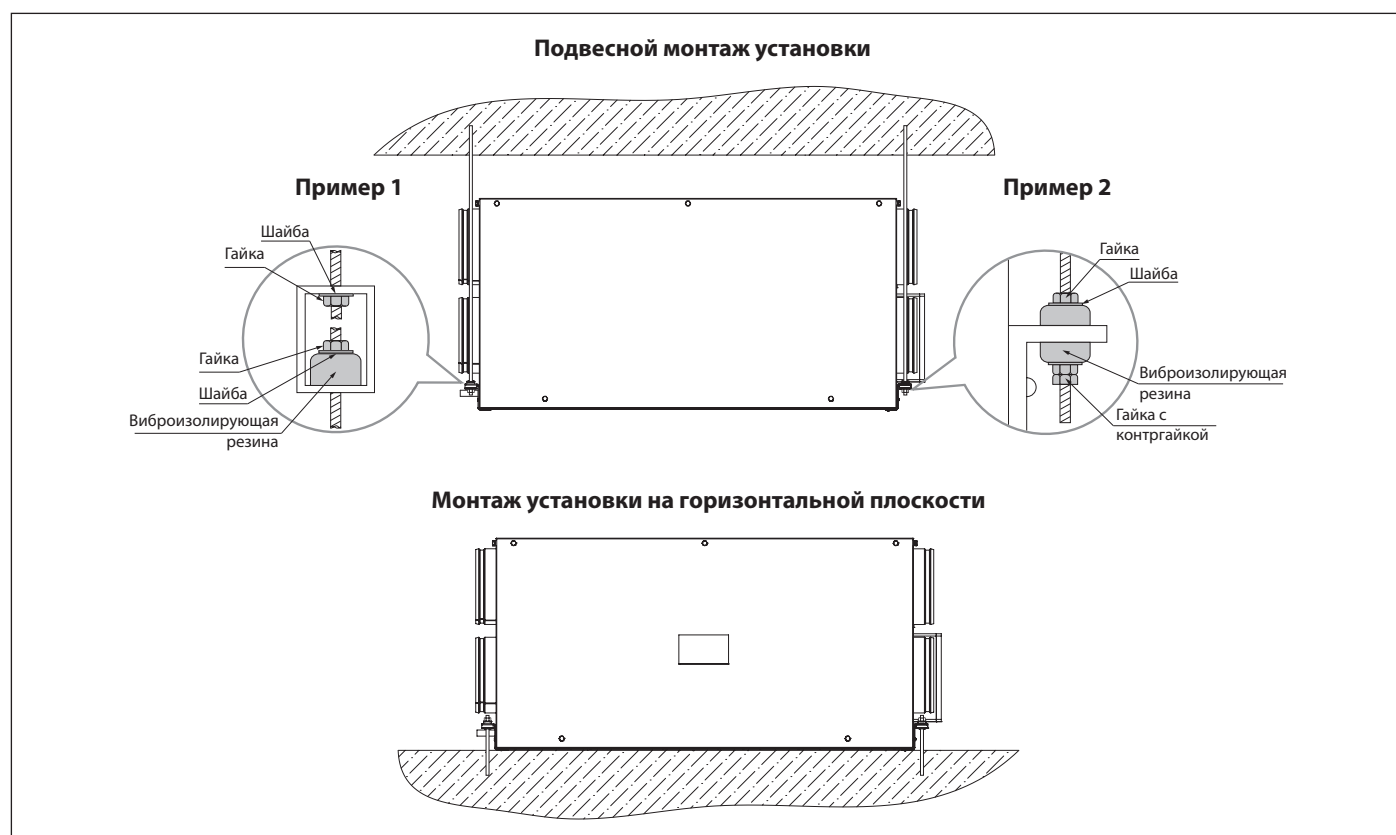
Рис. 6. Монтаж
