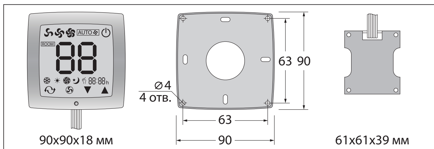
Рис. 12. Габаритные размеры панели управления
