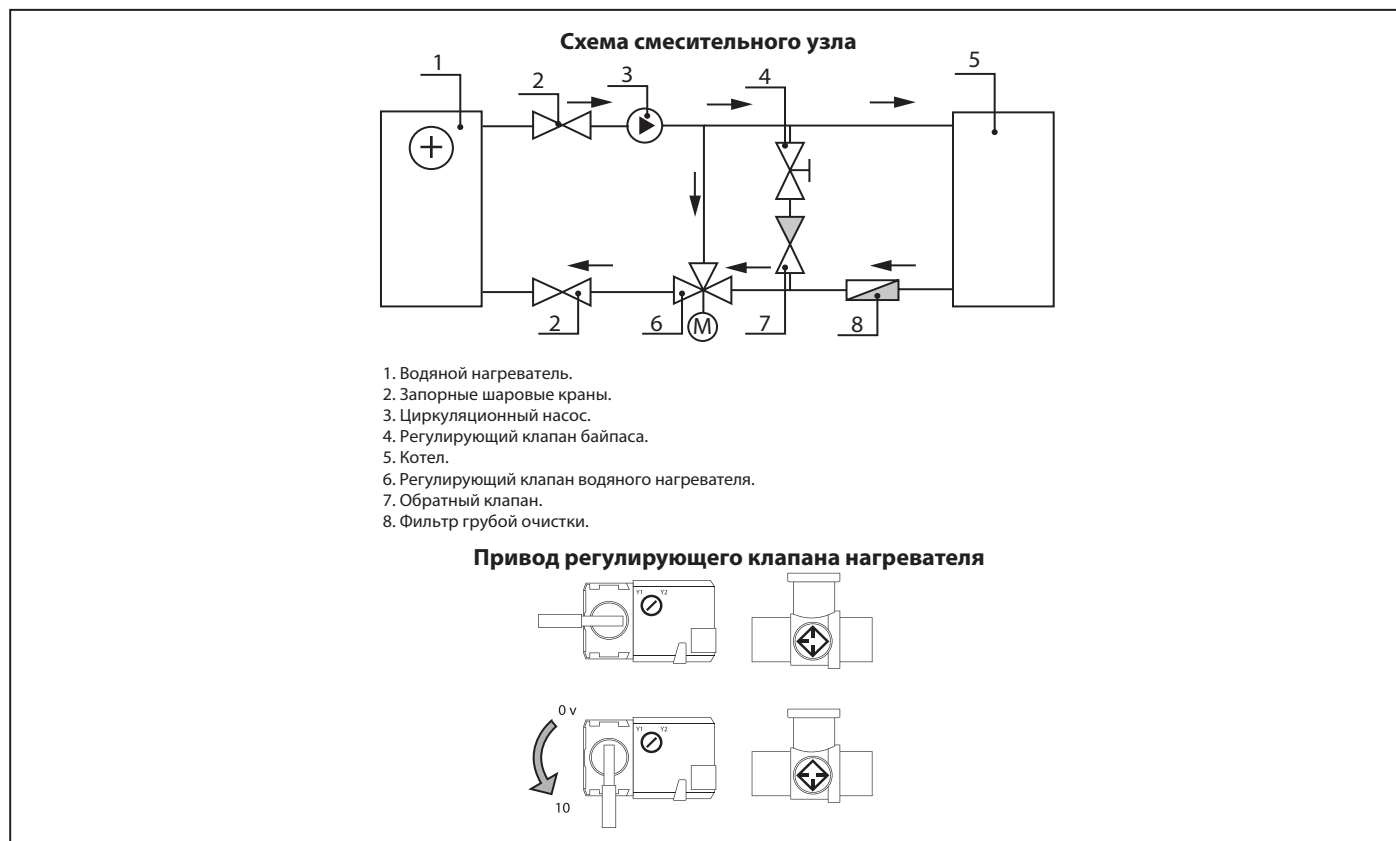
Рис. 8. Схема смесительного узла
