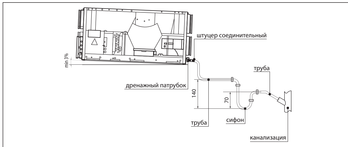
Рис. 9. Отвод конденсата
