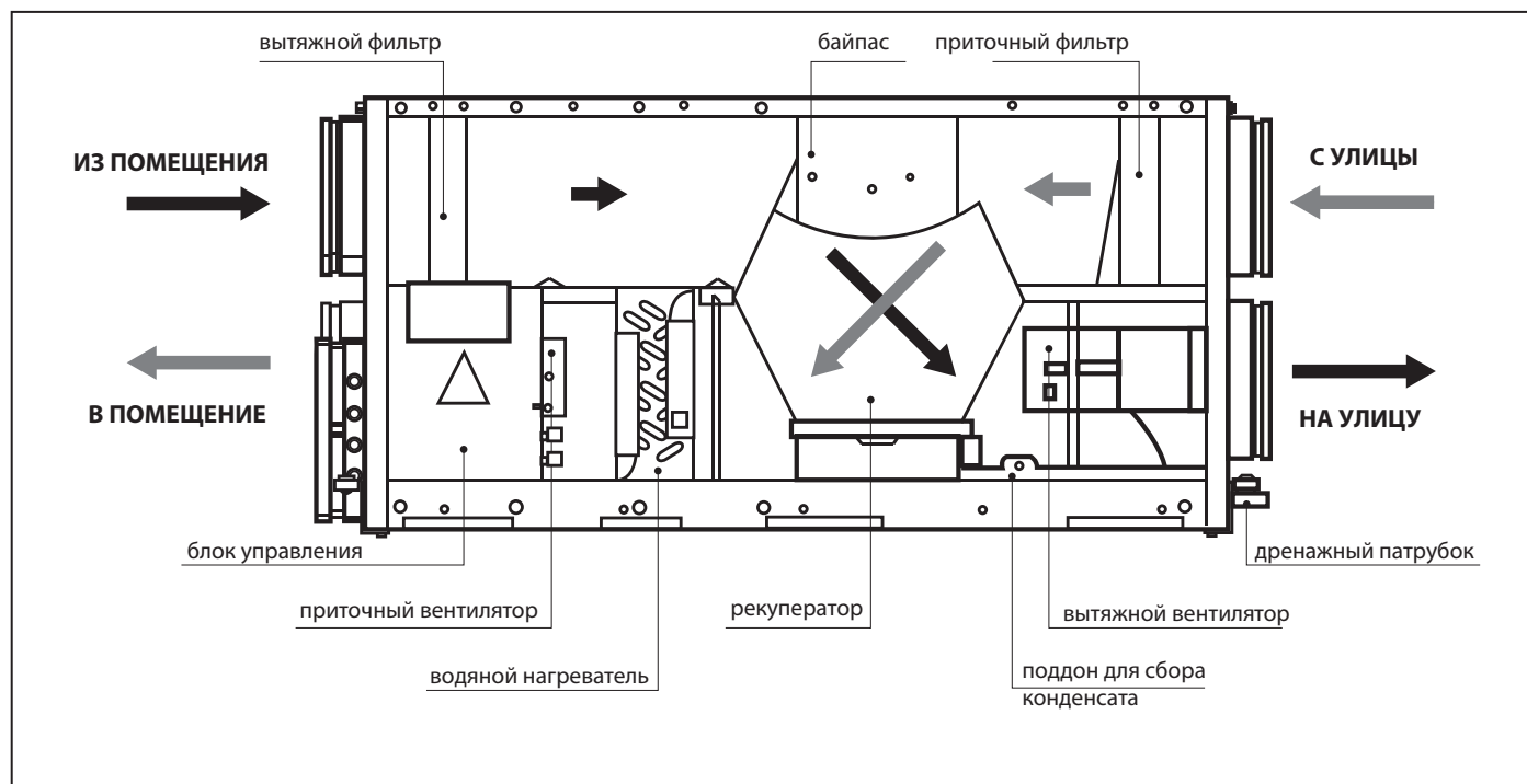
Рис. 1. Устройство и принцип работы
