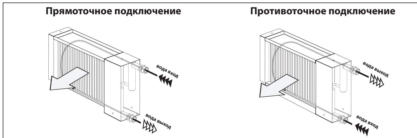
Рис. 7. Подключение водяного нагревателя
