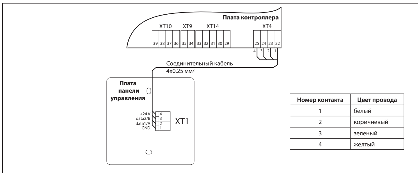
Рис. 9. Схема подключения панели управления
