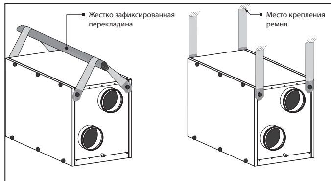
Рис. 5. Подвесной монтаж
