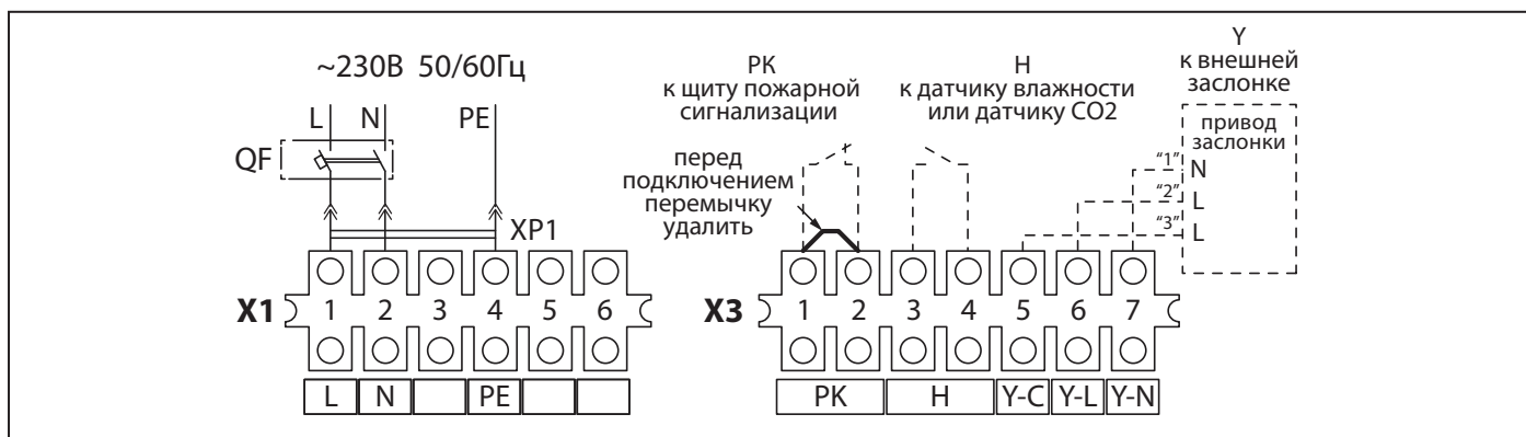
Рис. 8. Схема внешних подключений
