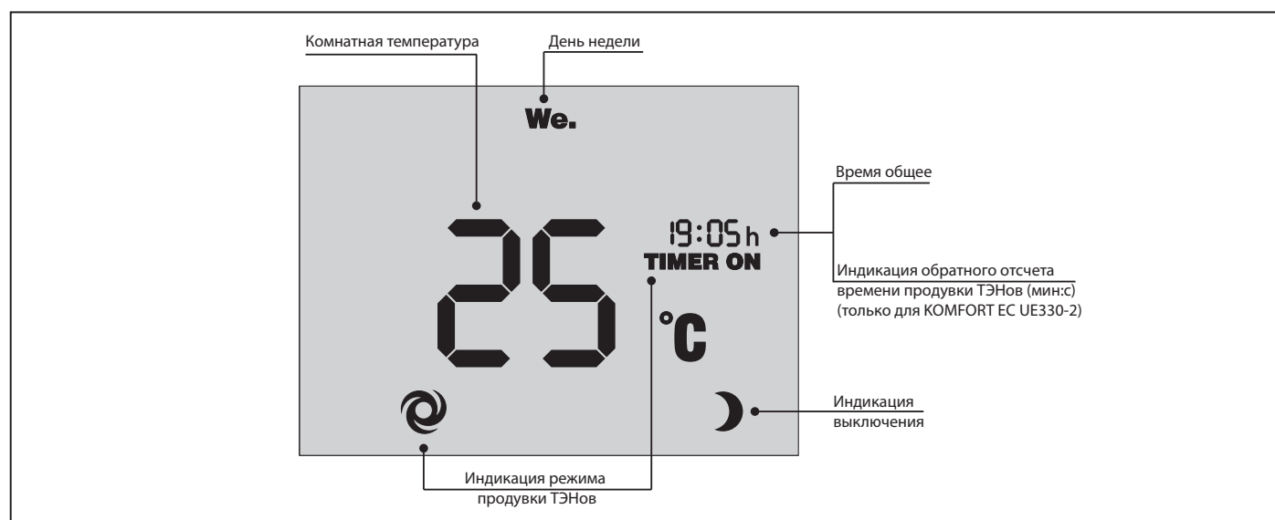
Рис. 9. Дисплей настенной панели управления в выключенном состоянии
