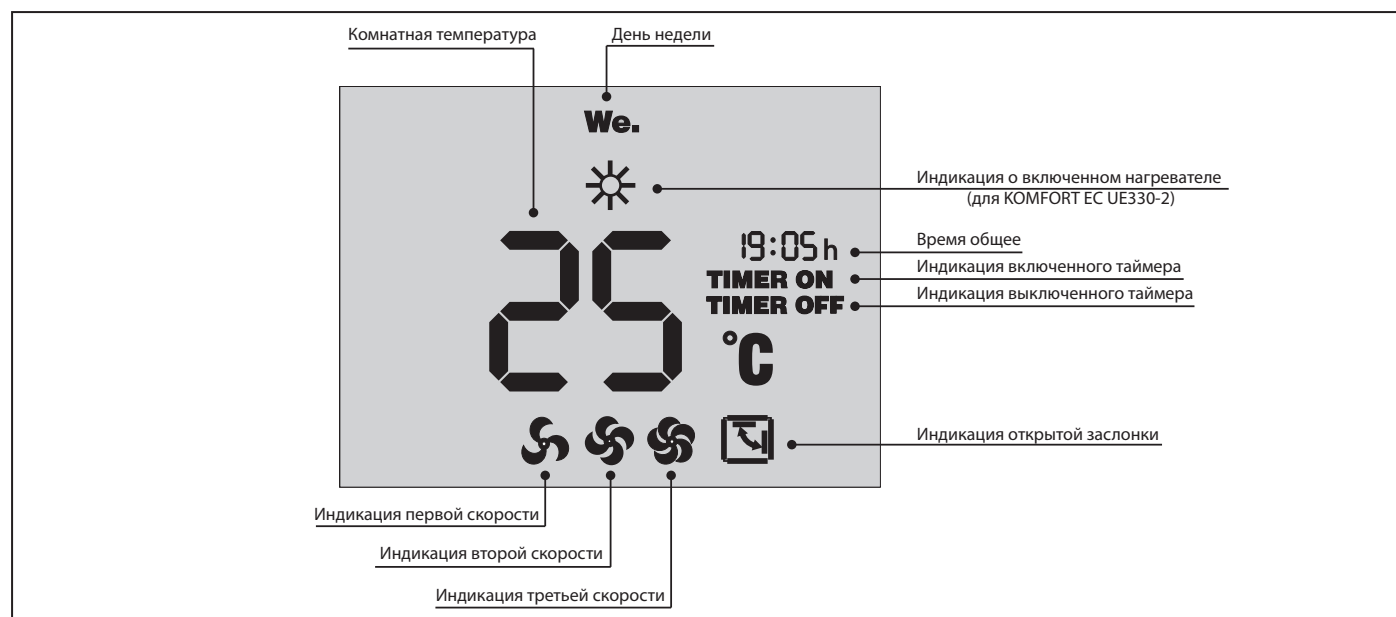
Рис. 10. Дисплей настенной панели управления во включенном состоянии
