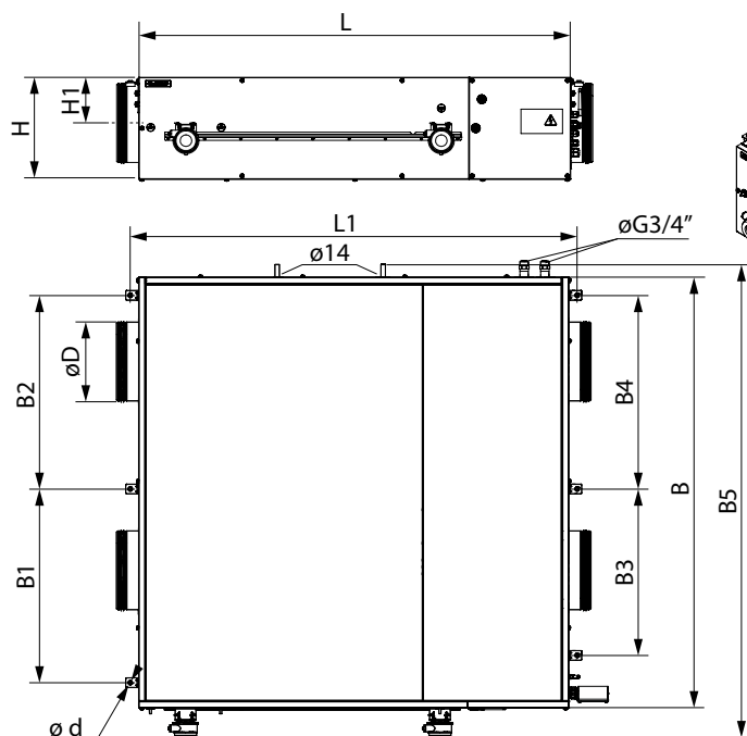
Размеры, мм
