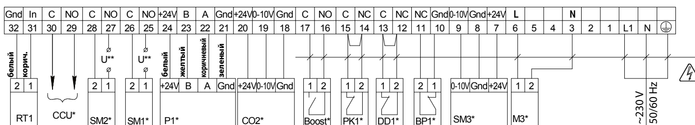
СХЕМА ВНЕШНИХ ПОДКЛЮЧЕНИЙ KOMFORT EC DBW 2000 S21
