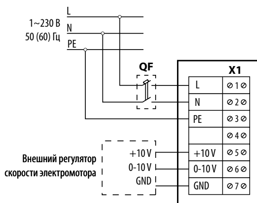
Схема электрических подключений
