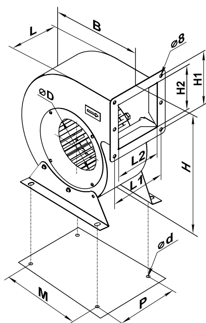
Габаритные размеры и варианты положения корпуса вентилятора Helix(-z)
