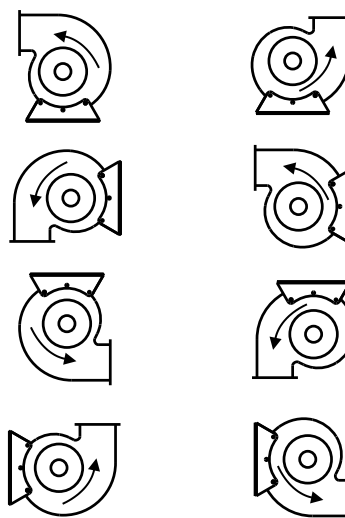
ВОЗМОЖНЫЕ ВАРИАНТЫ ПОЛОЖЕНИЯ КОРПУСА ВЕНТИЛЯТОРА Helix(-z) (вид со стороны притока воздуха)
