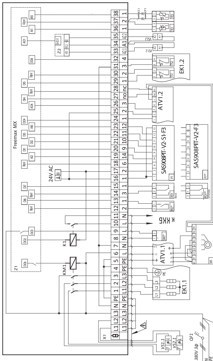
Схема внешних подключений BLAUBOX DE1300-12 Pro, BLAUBOX DE2500-18 Pro, BLAUBOX DE3300-21 Pro
