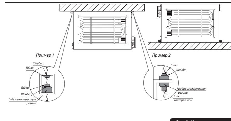
Рис. 3. Монтаж установки
